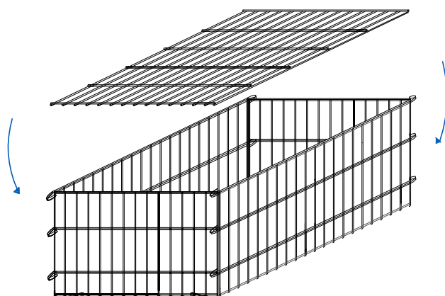
couvercle
