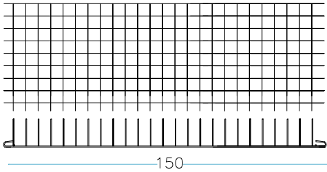
nr. 2 pz. latérales longs 150 x H. 50 cm
