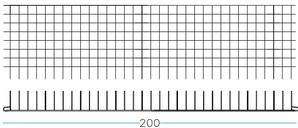
nr. 2 pc. latérales longs 200 x H. 50 cm
