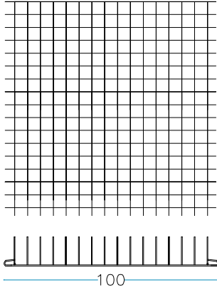
nr. 2 pc. Long side panel 100 x H. 100 cm
