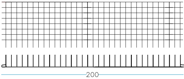
nr. 2 pc. Long side panel 200 x H. 50 cm
