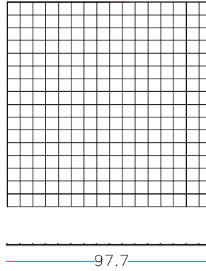
nr. 2 pc. Short side panel 100 x H.100 cm
