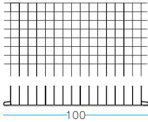
nr. 2 pc. Long side panel 100 x H. 50 cm
