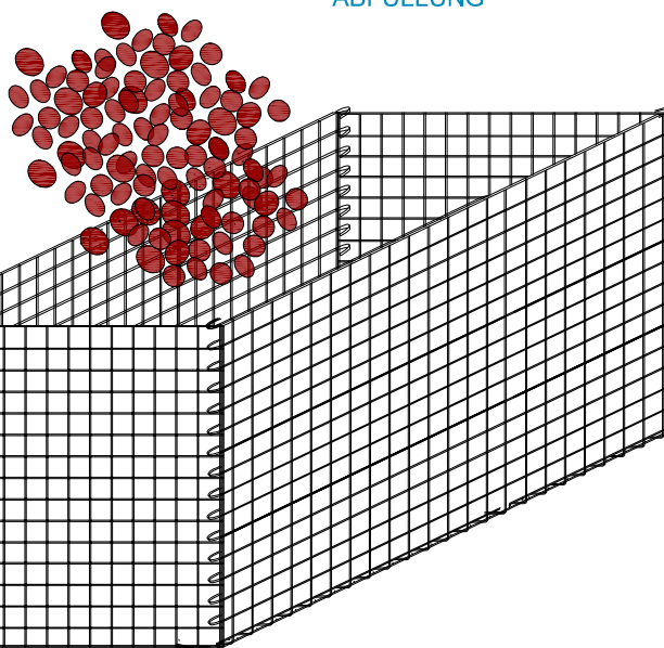
STEP 13 ABFÜLLUNG
