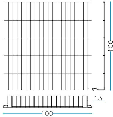
nr. 2 Stck. Längs Seite 100 x H. 100 cm
