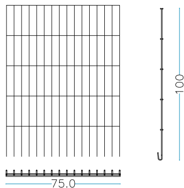
nr. 2 Stck. Kopf Seite 75 x H.100 cm
