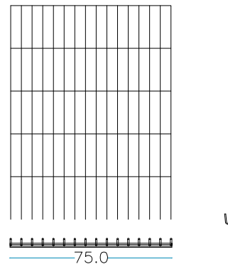
nr. 2 Stck. Kopf Seite 75 x H. 100 cm
