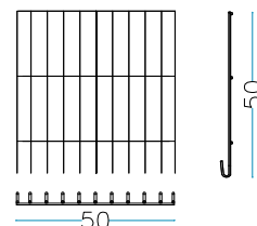
nr. 2 Stck. Kopf Seite 50 x H. 50 cm
