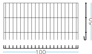
nr. 2 Stck. Kopf Seite 100 x H. 50 cm
