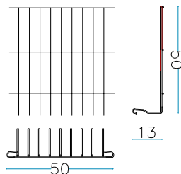
nr. 2 pc. Long sides 50 x H. 50 cm
