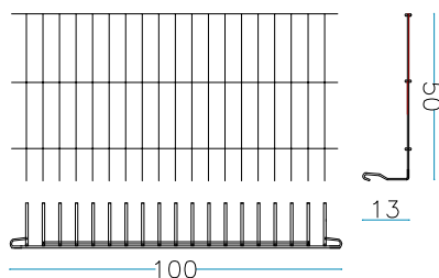
nr. 2 Stck. Längs Seite 100 x H. 50 cm
