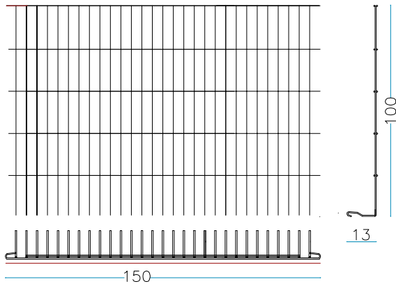
nr. 2 Stck. Längs Seite 150 x H. 100 cm
