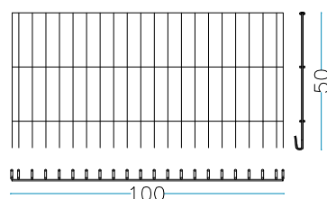
nr. 2 Stck. Kopf Seite 100 x H. 50 cm
