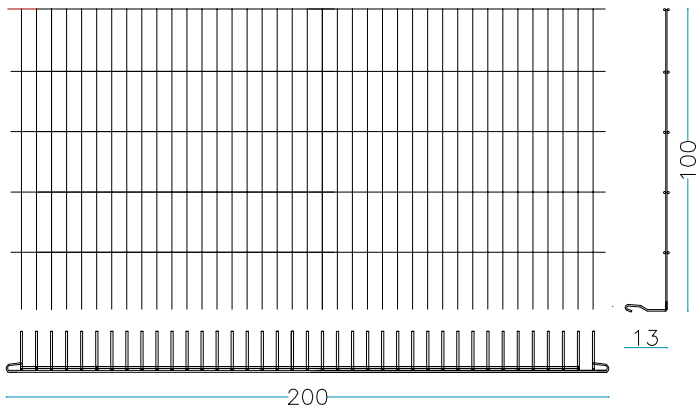
nr. 2 Stck. Längs Seite 200 x H. 100 cm
