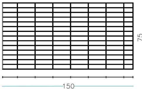
nr. 1 Stck. Boden 150 x 75 cm
