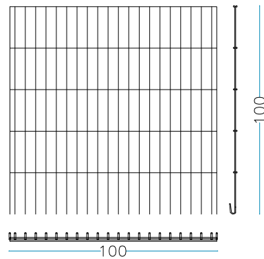
nr. 2 Stck. Kopf Seite 100 x H. 100 cm
