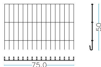
nr. 2 Stck. Kopf Seite 75 x H. 50 cm
