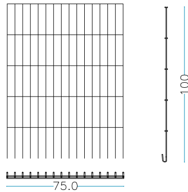
nr. 2 Stck. Kopf Seite 75 x H.100 cm
