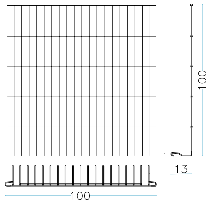
nr. 2 Stck. Längs Seite 100 x H. 100 cm
