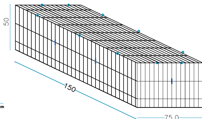
nr. 1 Querstreben L. 150 cm.
