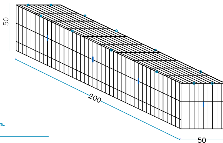
nr. 3 Querstreben L. 50 cm.
