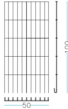
nr. 2 Stck. Kopf Seite 100 x H.100 cm
