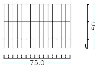
nr. 2 Stck. Kopf Seite 75 x H. 50 cm
