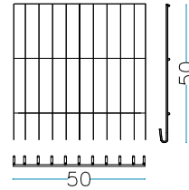
nr. 2 Stck. Kopf Seite 100 x H. 50 cm
