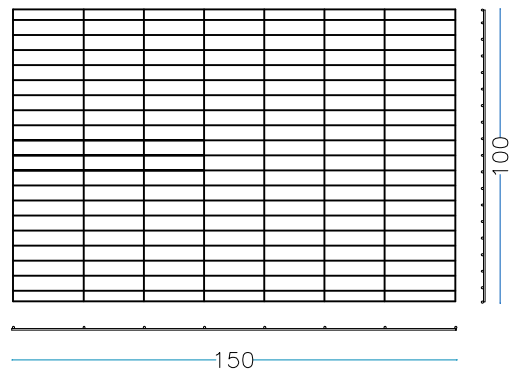
nr. 1 Stck. Deckel 150 x 100 cm
