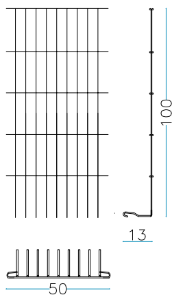
nr. 2 pc. Long sides 50 x H. 50 cm
