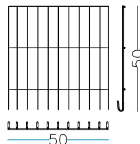
nr. 2 Stck. Kopf Seite 50 x H. 50 cm
