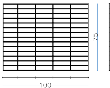
nr. 1 Stck. Boden 100 x 75 cm
