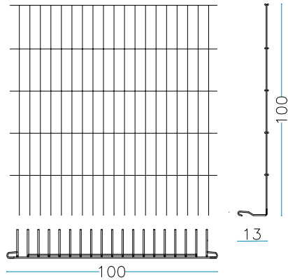
nr. 1 Stck. Boden 100 x 100 cm
