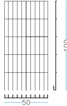
nr. 2 Stck. Kopf Seite 50 x H.100 cm
