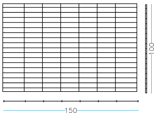
nr. 1 Stck. Boden 150 x 100 cm
