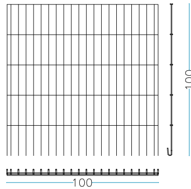
nr. 2 Stck. Kopf Seite 100 x H. 100 cm
