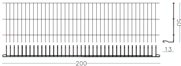
nr. 2 Stck. Längs Seite 150 x H. 50 cm
