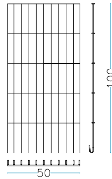
nr. 2 Stck. Kopf Seite 50 x H.100 cm
