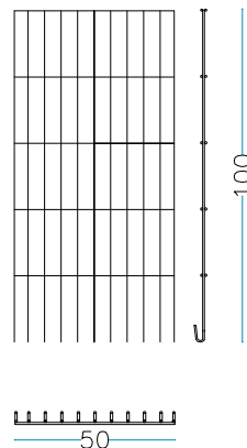
nr. 2 pc. Short sides 50 x H. 50 cm
