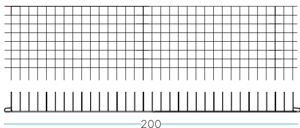
nr. 2 pz. Längs Seite 200 x H. 50 cm
