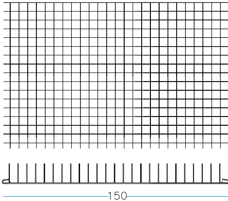
nr. 2 Stck. Längs Seite 150 x H. 100 cm
