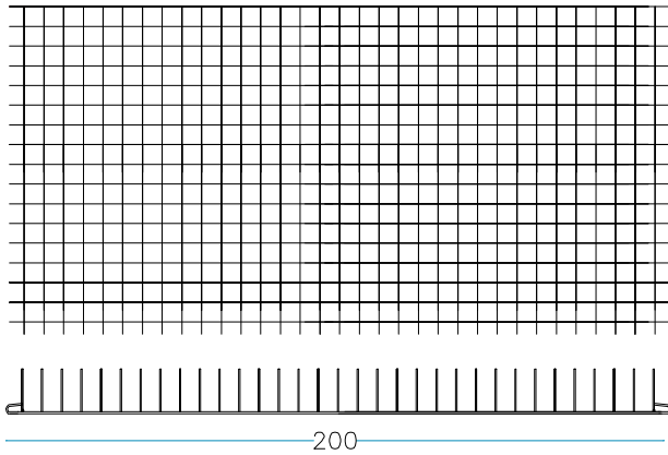
nr. 2 pz. Boden Deckel 200 x 100 cm
